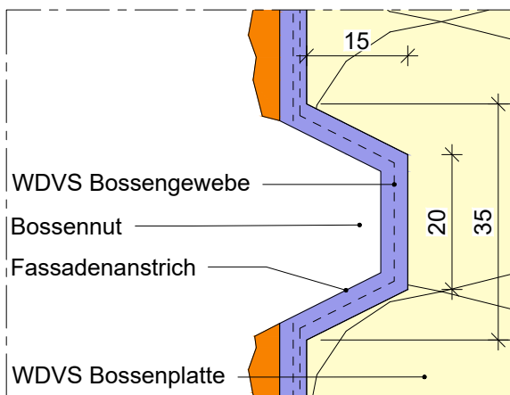
Trapeznut breit (TB) M 1:1
