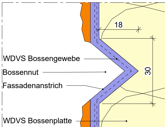
Dreiecksnut (DN) M 1:1
