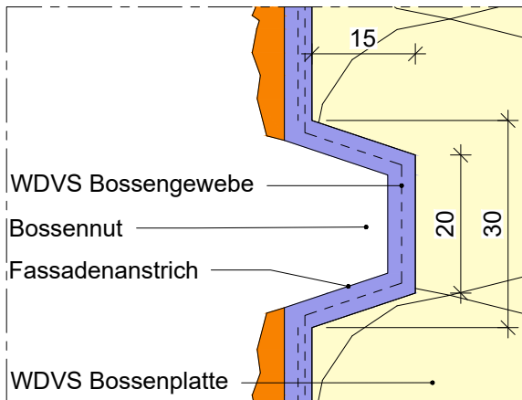
Trapeznut schmal (TS) M 1:1
